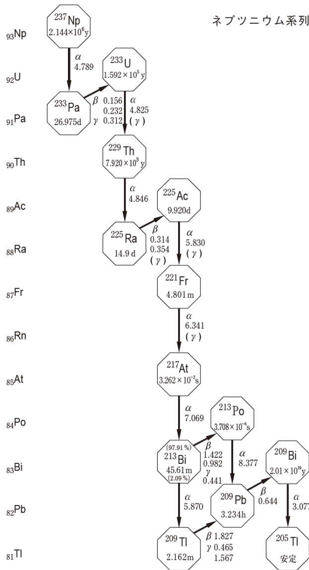
図 2 - 1 ^{225}\text{Ac} の放射性壊変
